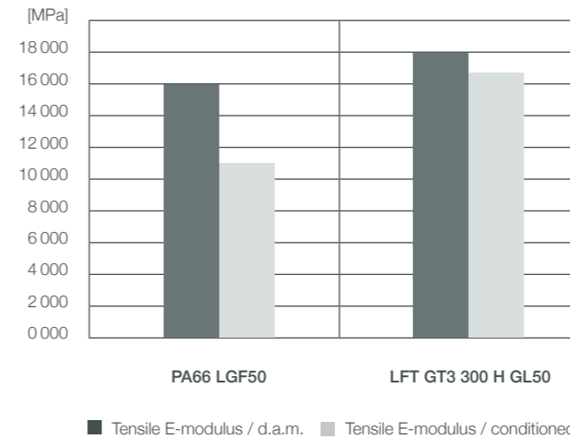
Comparison Tensile E-modulus (ISO 527)
